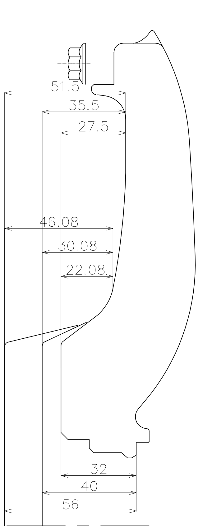
P.C.D. 100~120
